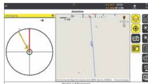
Abstecken eines Punktes
